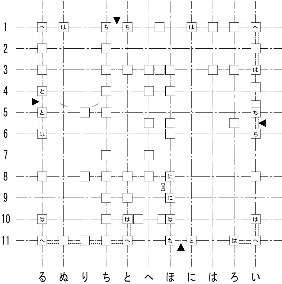
1 階柱壁伏図
