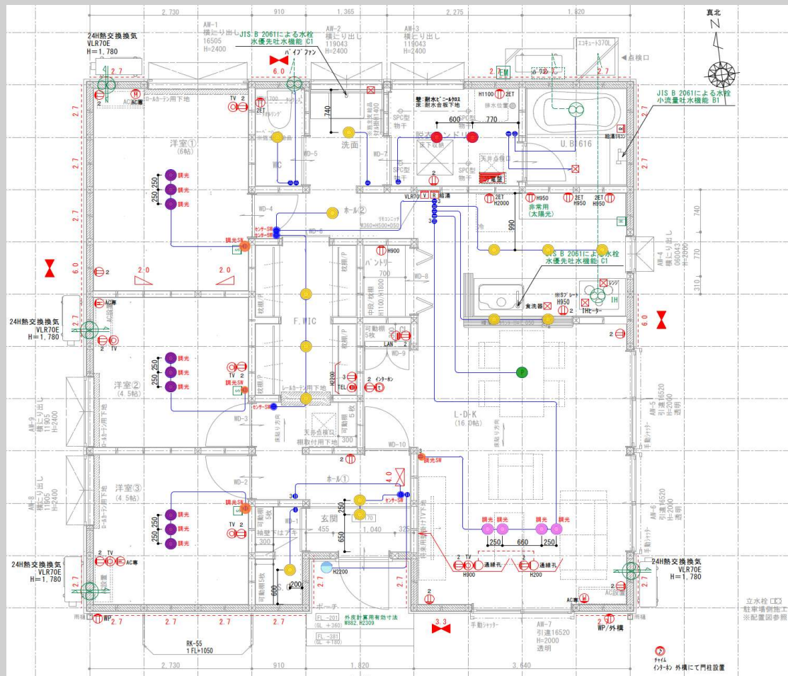
1階
